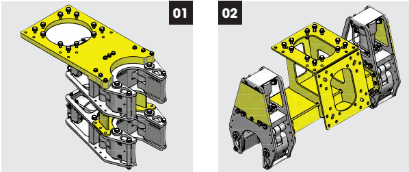
01 Vertikale Ausrichtung Klemmzangen // vertical alignment of the clamps 02 Horizontale Ausrichtung Klemmzangen // horizontal alignment of the clamps
