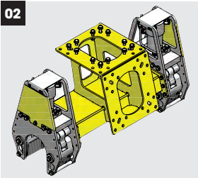
01 Vertikale Ausrichtung Klemmzangen // vertical alignment of the clamps 02 Horizontale Ausrichtung Klemmzangen // horizontal alignment of the clamps
